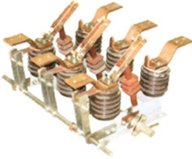
قاطع خارجي بدون حمل Off load outdoor disconnector
