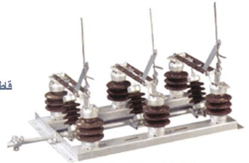
قاطع خارجي بقرون تفرغ Outdoor switch disconnector (Whips)
