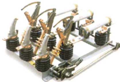
قاطع داخلي على الحمل On load indoor switch disconnector
