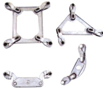
مخمدات خاصة لنواقل الشبكة الهوائية Spacer dampers
